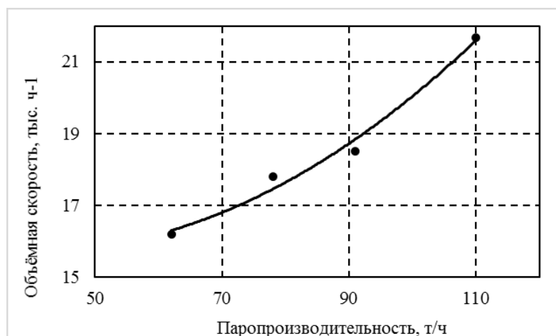
Рисунок 4 – Зависимость объемной скорости дымовых газов в сечении блока катализатора от нагрузки котлоагрегата
