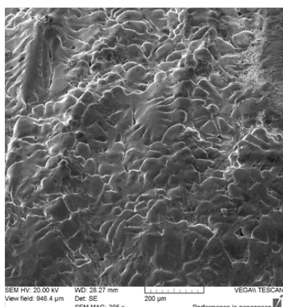
Рисунок 3 – Морфология поверхности на шарообразных алюминиевых оплавлениях после теплового разгона литий-ионного аккумулятора при 25% заряде батареи
