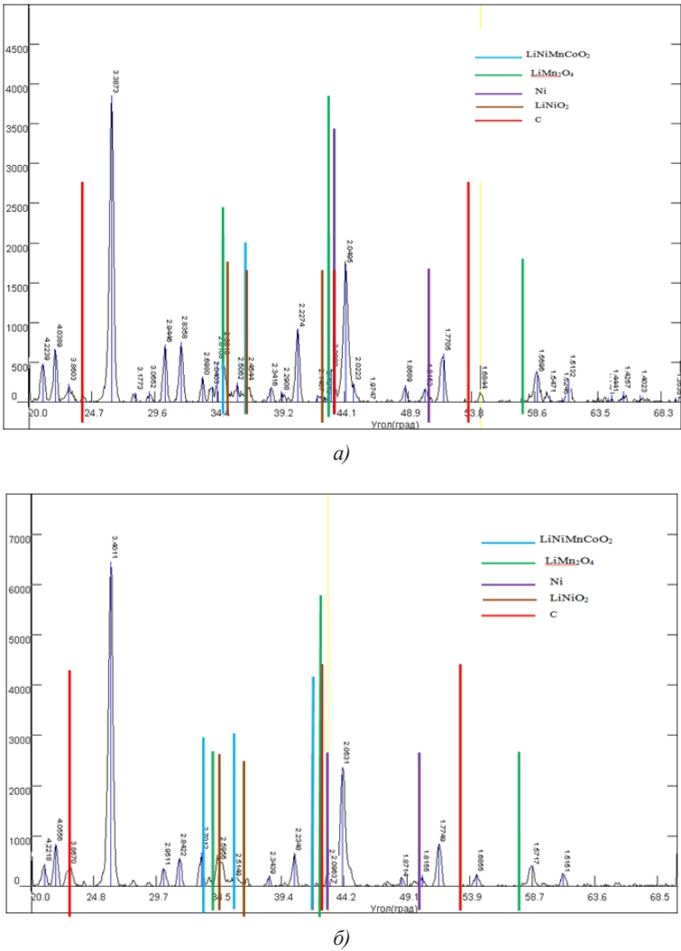
Рисунок 4 – Дифрактограммы внутреннего содержимого фрагментов исследуемых аккумуляторов: а, б – образцы 4-5
