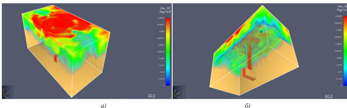
Рисунок 3 – Результаты моделирования распространения водородсодержащего газа при аварийной утечке из технологического трубопровода, находящегося под давлением, на 60 секунде: а); вид сверху; б) вид снизу
