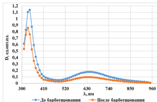
Рисунок 4 – Спектры триэтаноламинового раствора с гидроксокарбонатом меди до и после барботирования
