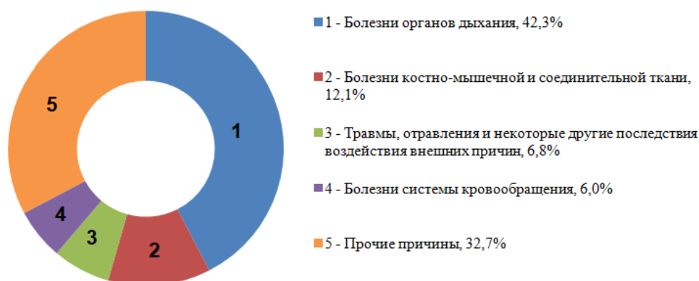
Рисунок 2 – Процентное распределение травм и заболеваний, приведших к временной нетрудоспособности работников предприятий по добыче полезных ископаемых (составлено авторами)
