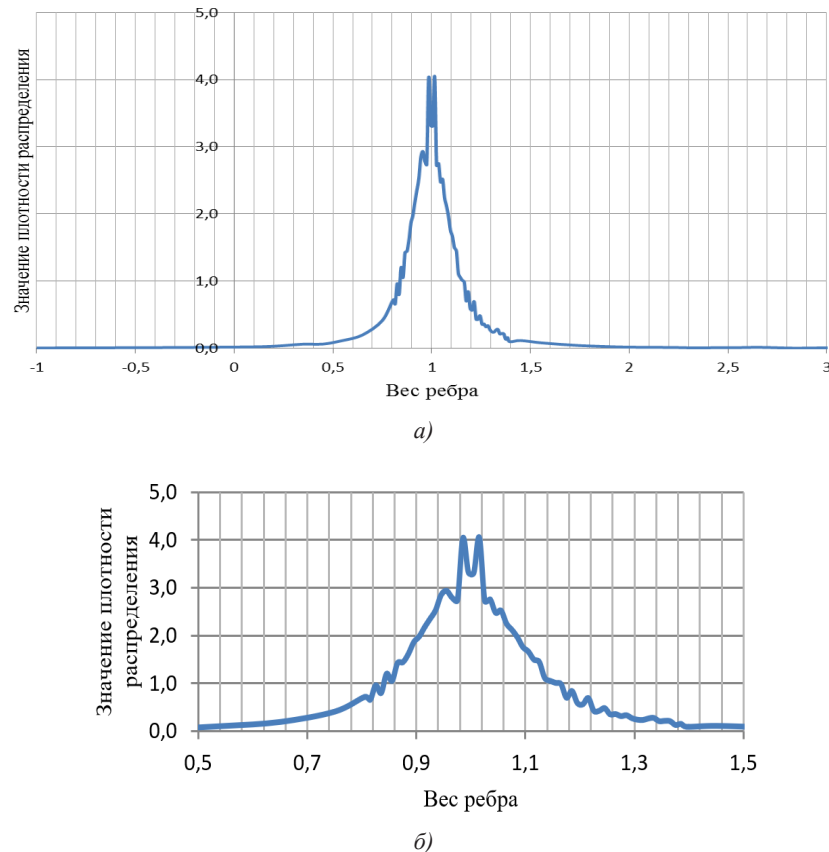
Рисунок 7 – Распределение весов для направления H_l в диапазоне от -1 до 3 (а) и в диапазоне от 0,5 до 1,5 (б)
