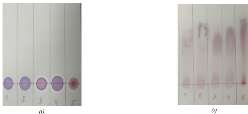
Рисунок 6 – Хроматограммы исходные (а) и после разделения (б): триэтаноламиновый раствор хлорида меди после продувки оксидом углерода (1,б) и без продувки (2,б); триэтаноламиновый раствор гидроксокарбоната меди после продувки (3,б) и без продувки (4,б); ализарин-комплексон (5)
