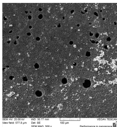
Рисунок 4 – Морфология поверхности на алюминиевой фольге после теплового разгона литий-ионного аккумулятора при 50% заряде батареи
