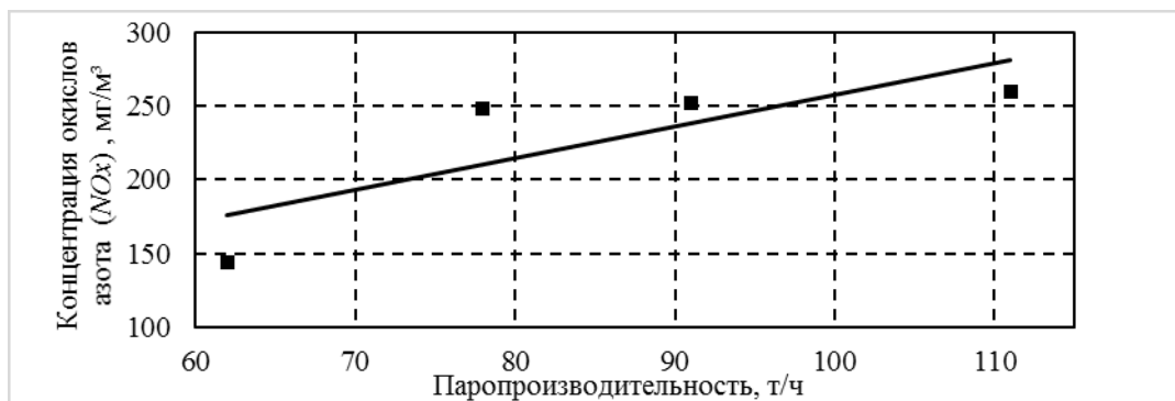
Рисунок 2 – Зависимость концентрации окислов азота в дымовых газах при варьировании нагрузки котла НЗЛ-110 (топливо – природный газ)
