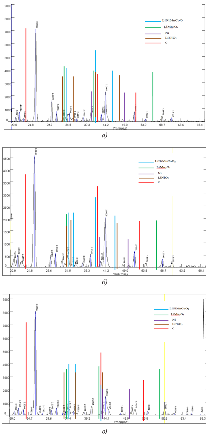
Рисунок 3 – Дифрактограммы внутреннего содержимого фрагментов исследуемых аккумуляторов: а, б, в – образцы 1-3
