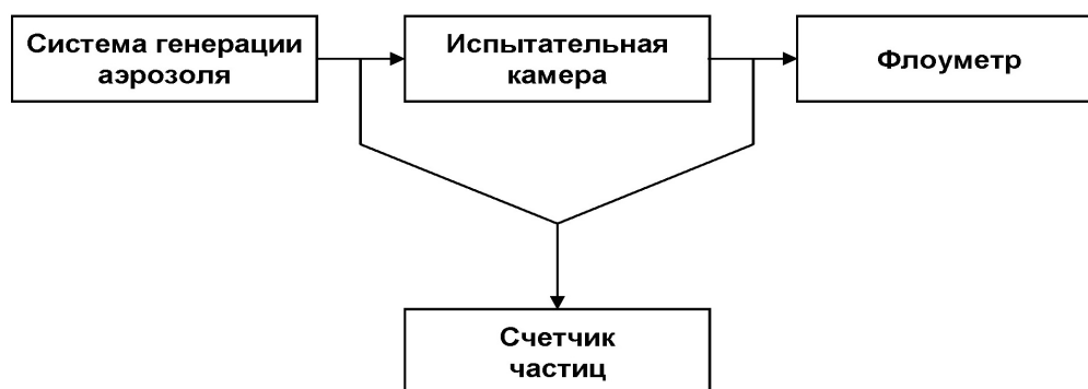
Рисунок 2 – Принципиальная схема установки для определения эффективности фильтрации наночастиц
