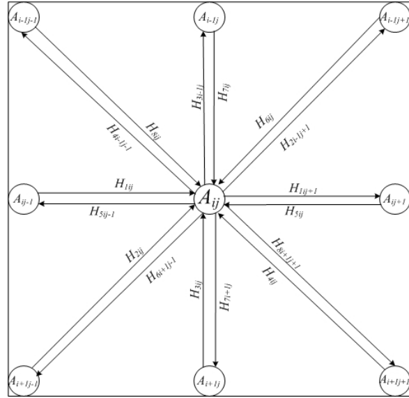
Рисунок 6 – Часть ориентированного графа: вершина A_{ij} инцидентные с ней ребра и смежные с ней вершины
