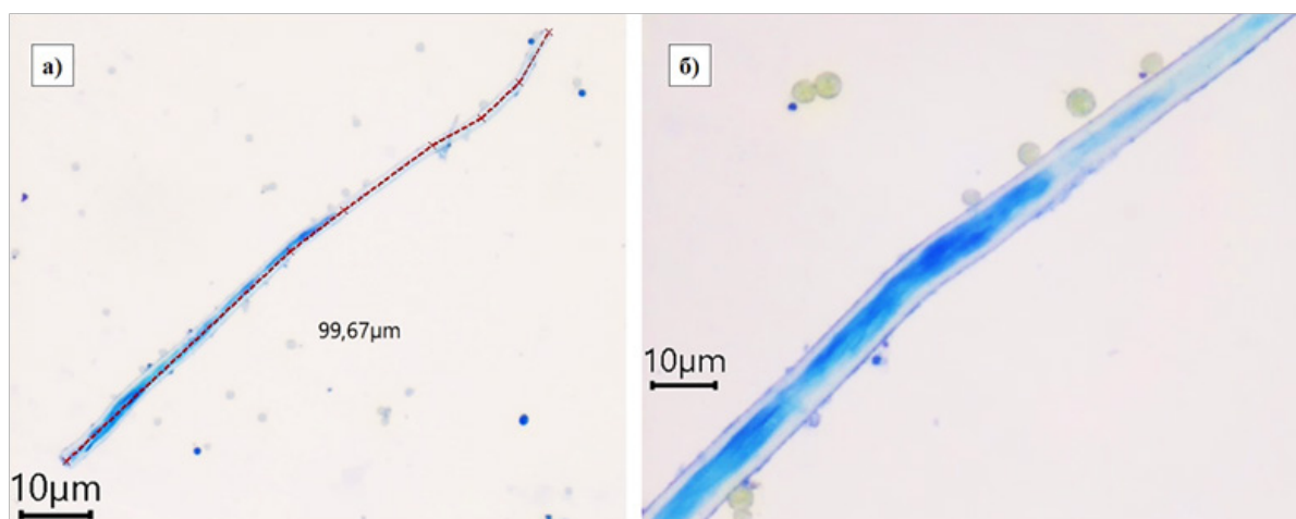
Рисунок 8 – Процесс гетероагрегации водорослей к частице микропластика на седьмые сутки:
