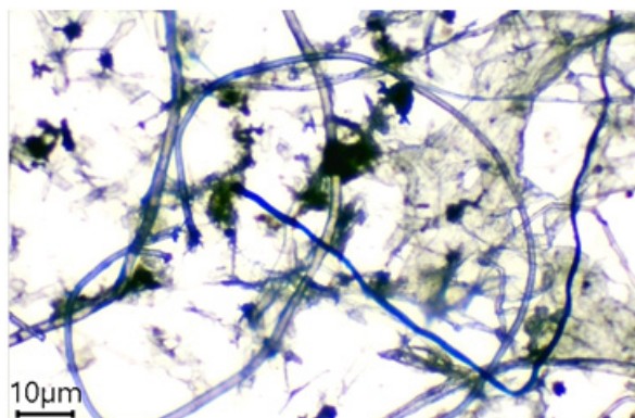
Рисунок 5 – Частицы микропластика, обнаруженные в пробе №3
