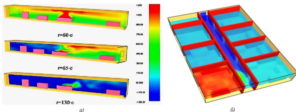
Рисунок 4 – Результаты компьютерного моделирования подавления пожара продувкой наружным воздухом при -400^{\circ}\text{C} , VB=10\text{ м/с} :
