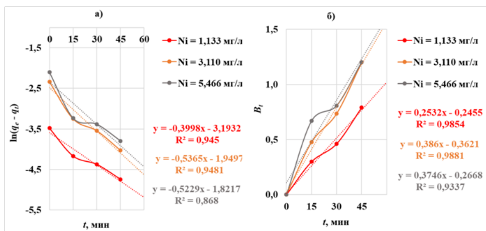
Рисунок 3 – Кинетические кривые сорбции в координатах уравнения: Бойда (а) для внешней (пленочной) диффузии; Бойда-Адамса-Майерса (б) для диффузии внутри адсорбента
