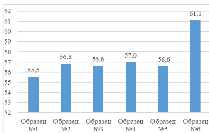
Рисунок 3 – Сравнительная диаграмма расчета температур перегрева различных композитных материалов
