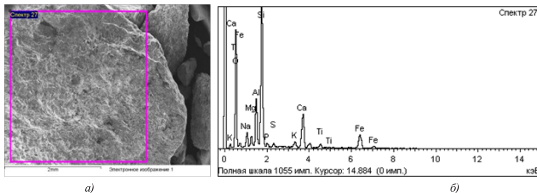
Рисунок 6 – Электронное изображение (а) с частицей сложного состава в шламе пробы Зкр, характеристический спектр (б), набранный по указанной площади в пределах частицы
