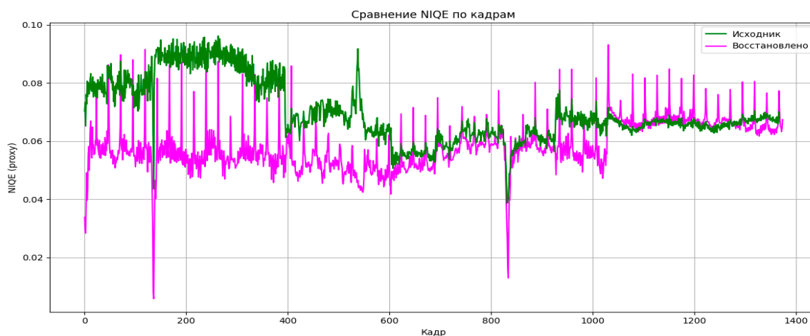
Рисунок 5 – Сравнение сканкопии материалов с преобладанием «маджента» (Исходник) и обработки программой «ЦветовоеВосстановление» (Восстановлено) по метрике NIQE (Показатель качества естественного изображения)
