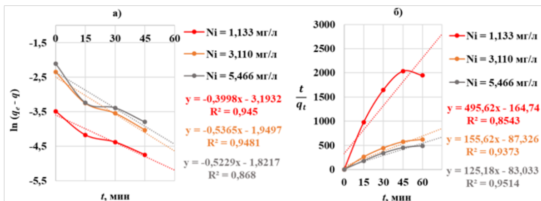
Рисунок 5 – Кинетические кривые в координатах уравнения: псевдо-первого порядка (а), псевдо-второго порядка (б)
