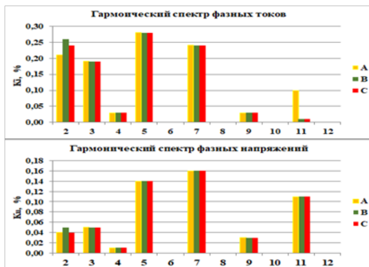
Рисунок 5 – Изменения коэффициентов гармонических искажений фазных токов и напряжений при радиальной несоосности вала синхронной машины СД-13-34-8, составляющей 0,5 мм
