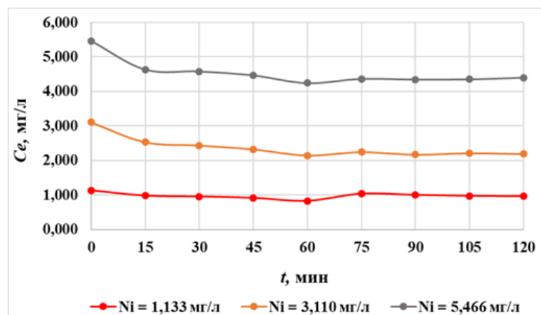
Рисунок 1 – Изменение концентрации адсорбтива C_e в модельном растворе с течением времени t
