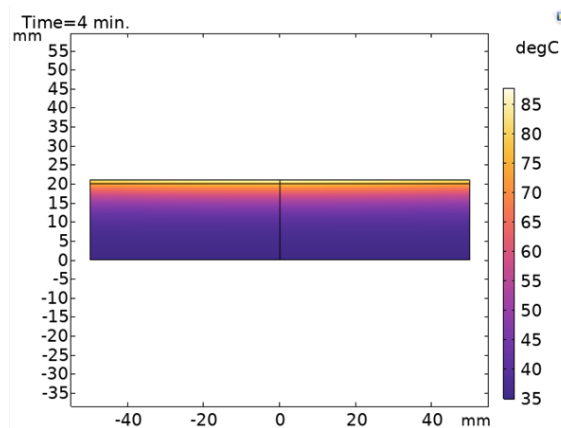
Рисунок 6 – Распределение температуры живой ткани в момент времени 4 минуты (керамика)
