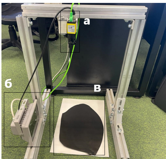
Рисунок 3 – Тестовая установка
