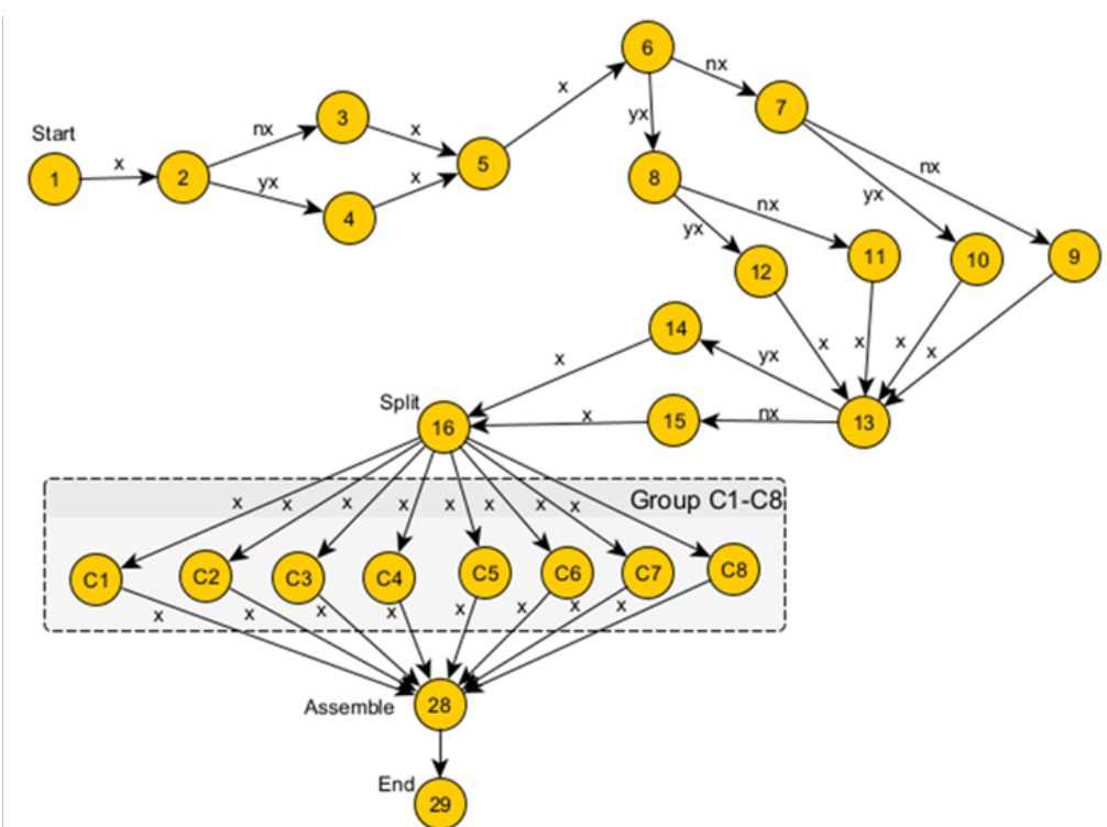
Рисунок 3 – Последовательно-параллельная сеть автоматов с вложенными состояниями Group C1-C8 выполнения приложения в кластере в режиме обработки SPMD (Single Program, Multiple Data)
