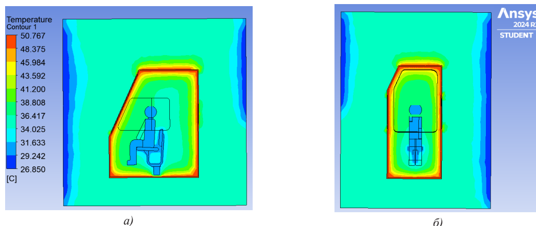
Рисунок 5 – Поля температуры ограждений кабины и воздуха внутри: а) вид сбоку, б) вид спереди
