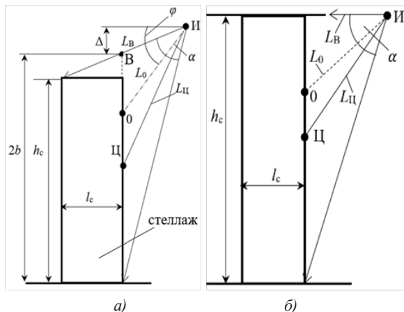
Рисунок 4 – Расчётные модели стеллажей (а – стеллаж не касается перекрытия, б – является опорой перекрытия). Обозначения: h_c , l_c – высота и ширина стеллажа; \alpha – угол раствора оросителя И; \varphi – угол наклона оси оросителя (для случая «б» \varphi=0,5\alpha ); 0 – точка пересечения оси оросителя с плоскостью стеллажа
