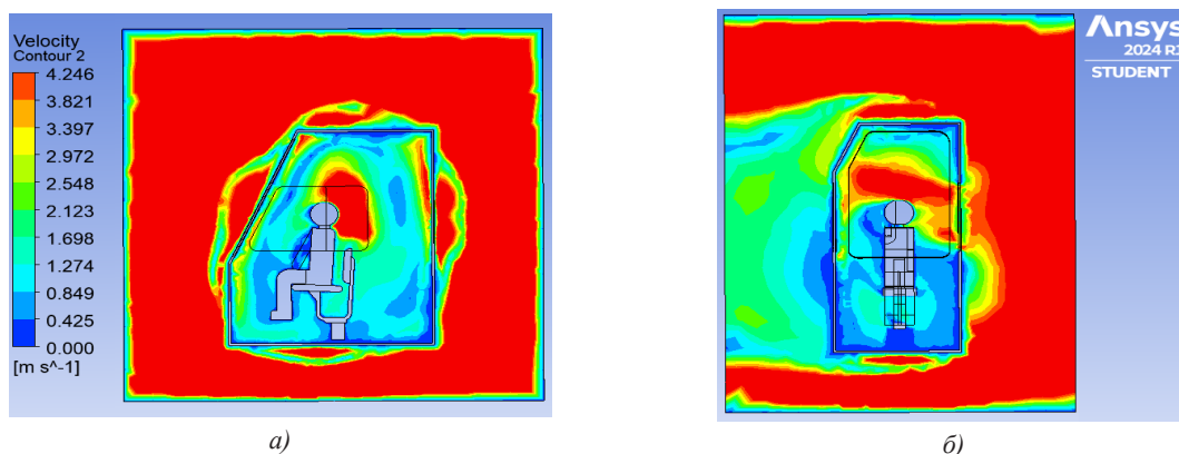
Рисунок 4 – Поля подвижности воздуха внутри кабины крана с открытой форточкой при боковом ветре 6,6 м/с: а) вид сбоку, б) вид спереди
