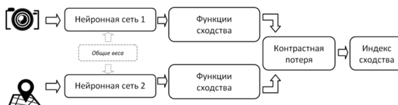
Рисунок 1 – Сиамская нейронная сеть
