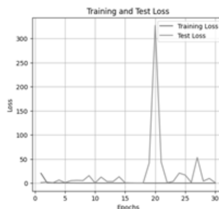
Рисунок 6 – График потерь во время обучения и тестирования по эпохам
