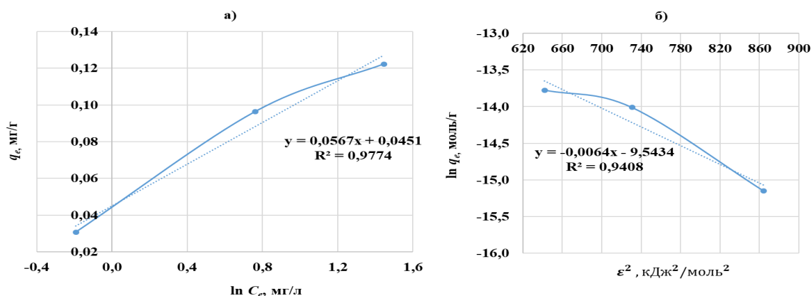
Рисунок 7 – Изотерма сорбции никеля в координатах уравнений: Холси (а) и Дубинина - Радушкевича (б)
