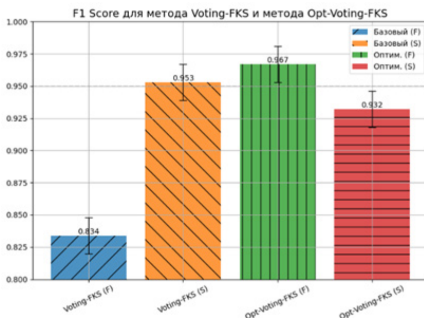
Рисунок 1 – График сравнения результатов работы оптимизированного ансамблевого метода Opt-Voting-FKS с контрольным методом Voting-FKS по метрике F1-Score
