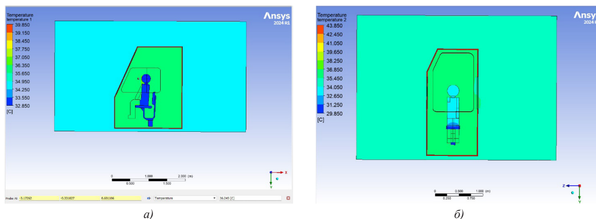
Рисунок 6 – Результаты моделирования при нагревающем микроклимате: а) вид сбоку, б) вид спереди
