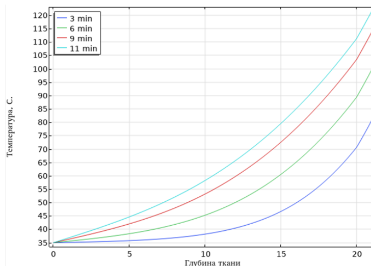
Рисунок 12 – Распределение температуры на разной глубине живой ткани в разные моменты времени (керамика)
