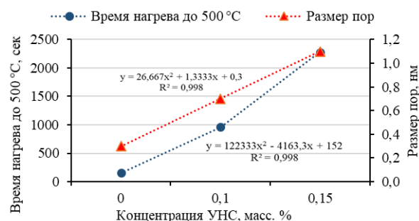
Рисунок 7 – Совмещенный график зависимости времени нагрева и размеров пор от диапазона концентраций УНС
