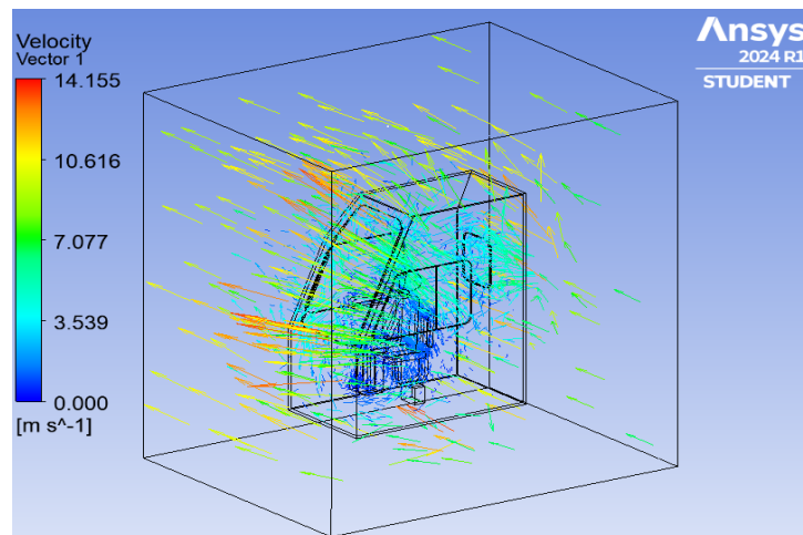
Рисунок 3 – Векторы движения воздуха в кабине железнодорожного крана с открытой форточкой окна при боковом ветре (3D)
