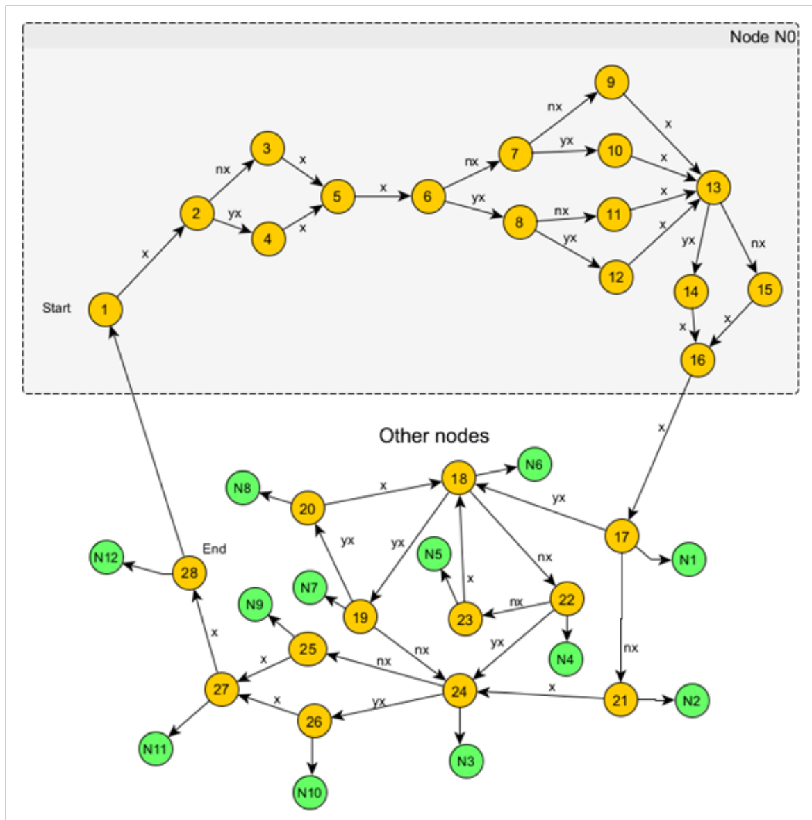
Рисунок 4 – Граф переходов состояний вычислительного кластера, соответствующий работе рас-пределенного многомодульного приложения в режиме MPMD (Multiple Programs, Multiple Data) на нижней части рисунка; верхняя часть соответствует последовательному подготовительному этапу
