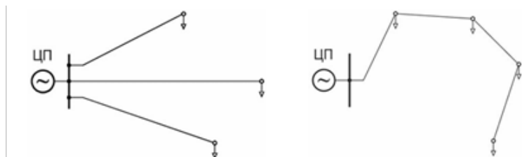
Рисунок 1 – Радиальная и магистральная конфигурации сети
