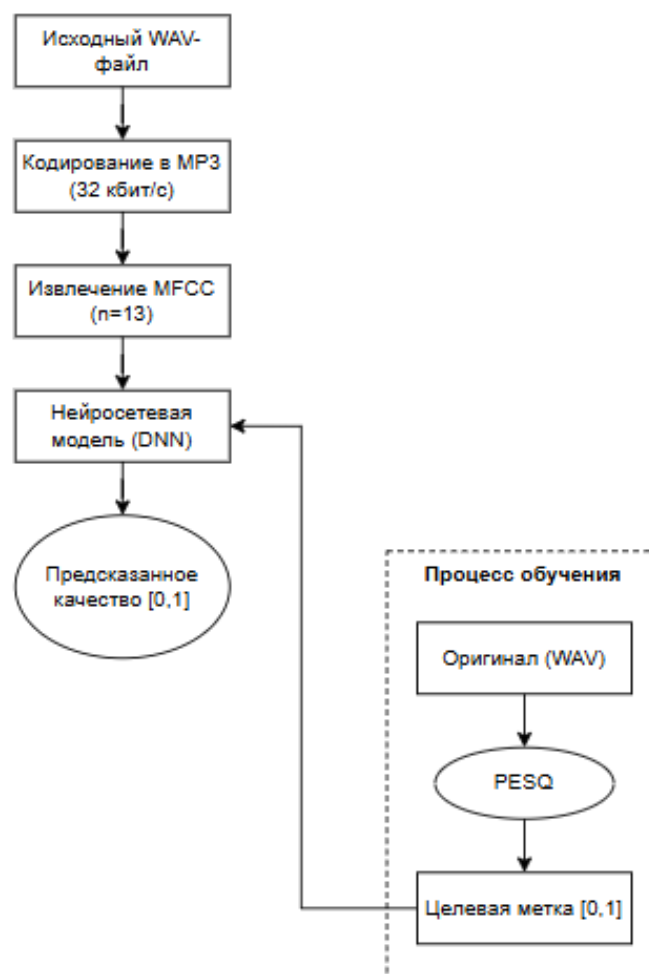
Рисунок 1 – Структура системы автоматического тестирования качества аудиокодеков на основе нейронных сетей
