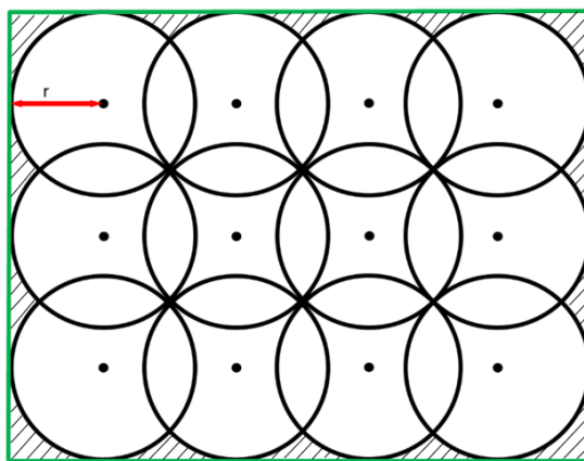
Рисунок 2 – Пример расположения видеокамер сеткой 4 на 3 внутри границ контролируемой площади ( N=4 , M=3 )
