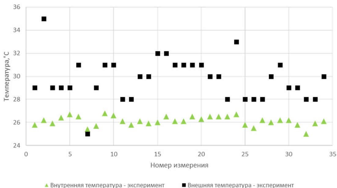
Рисунок 8 – Сравнение внешней и внутренней температуры по результатам экспериментальных исследований для теплого периода года
