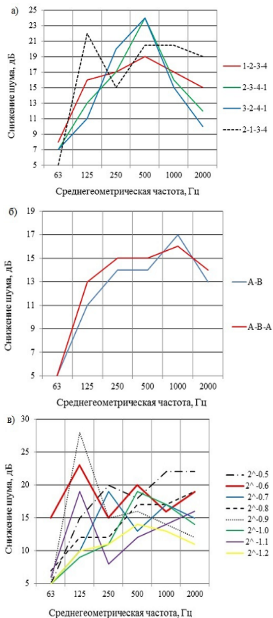
Рисунок 3 – Акустические характеристики щелевых устройств;
