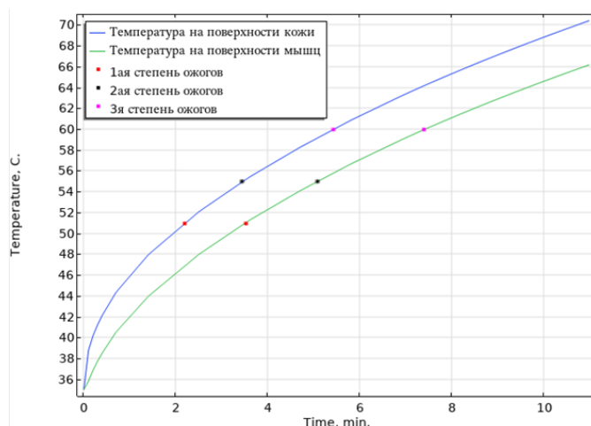
Рисунок 11 – Температура поверхности кожи и мышечной ткани от времени при нагреве от пламени углеводородов
