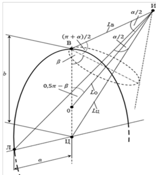
Рисунок 5 – Расчётная схема для зоны орошения в изометрии
