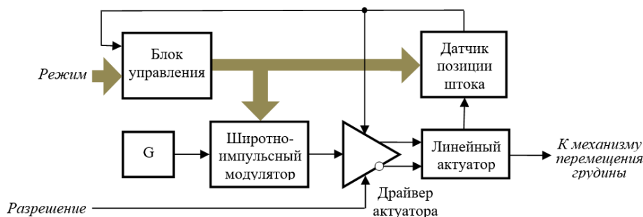
Рисунок 1 – Структурная схема имитатора дыхания
