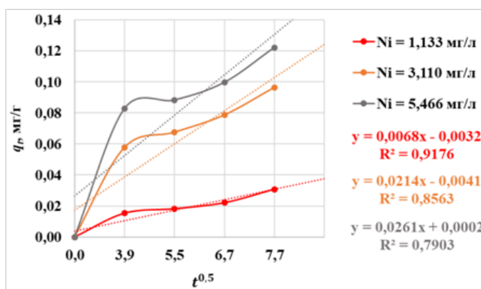
Рисунок 4 – Кинетические кривые сорбции в координатах уравнения Вебера-Морриса
