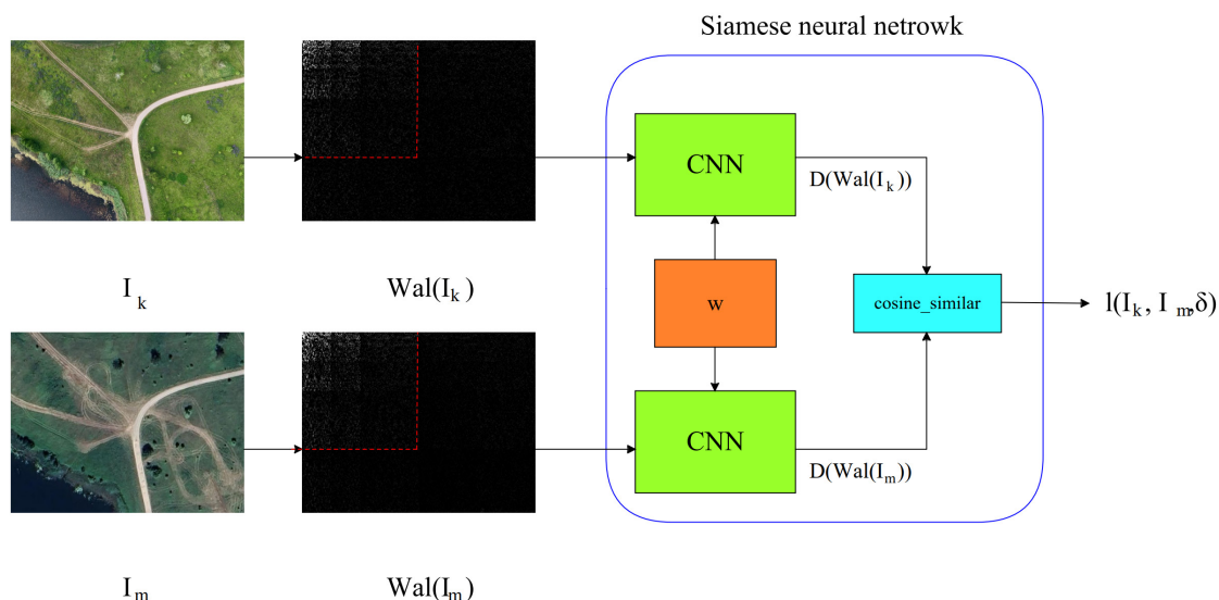
Рисунок 3 – Структурная схема модуля вычисления сходства с использованием сиамских сетей
