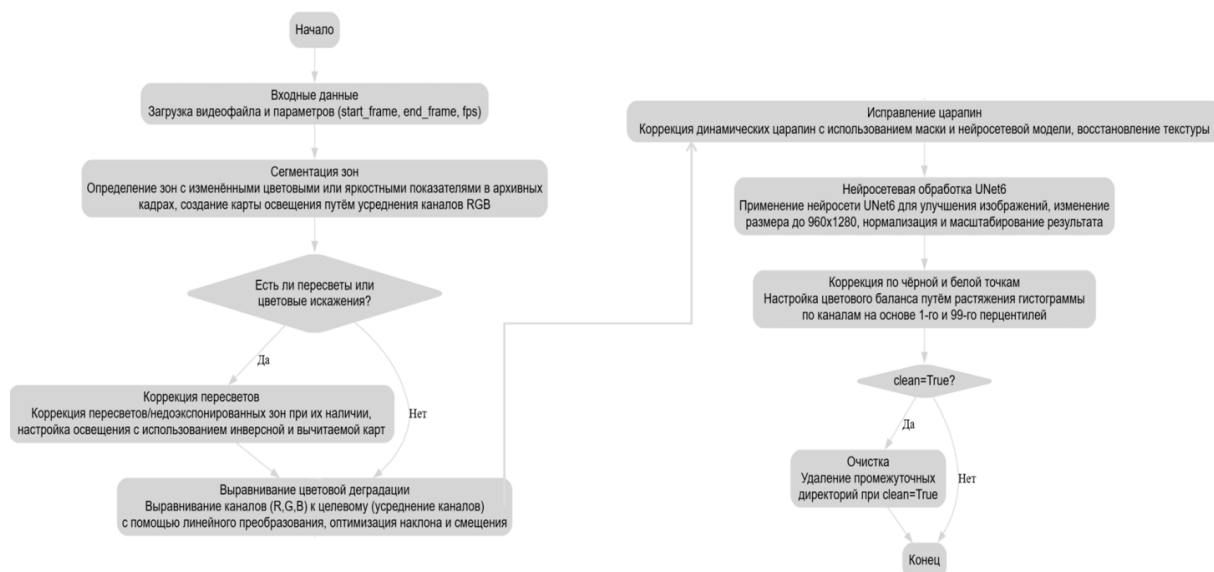
Рисунок 1 – Блок-схема работы программы «Цветовое восстановление»
