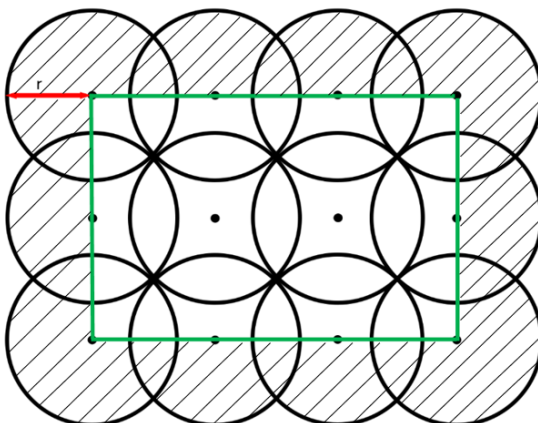
Рисунок 3 – Пример расположения видеокамер сеткой 4 на 3 ( N=4 , M=3 ) с расстановкой наружных видеокамер по периметру контролируемой площади
