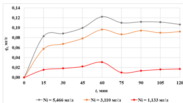
Рисунок 2 – Кинетическая кривая сорбции ионов Ni^{2+}
