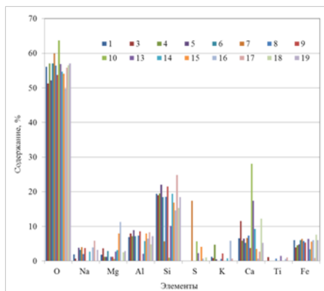
Рисунок 7 – Содержание элементов по спектрам пробы 1кр
