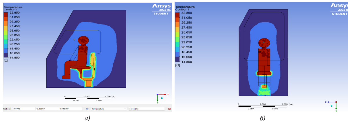
Рисунок 7 – Результаты моделирования температуры внутри кабины при 15°C окружающей среды: а) вид сбоку, б) вид спереди
