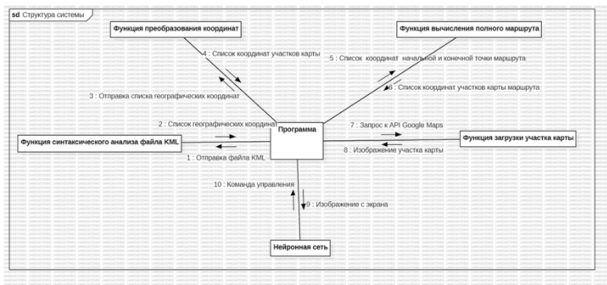
Рисунок 3 – Диаграмма взаимодействия навигационной системы
