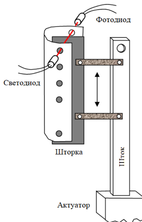
Рисунок 2 – Оптический датчик перемещения штока актуатора
