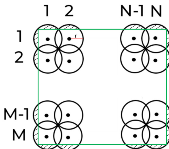
Рисунок 5 – Схема рационального расположения видеокамер на контролируемой территории (в общем виде)
