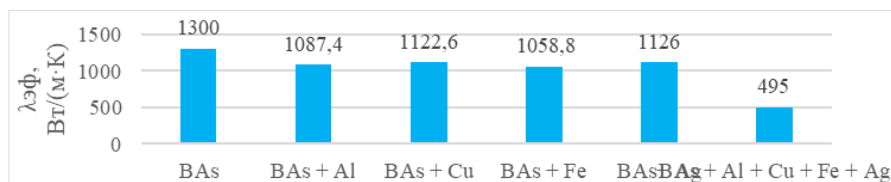
Рисунок 1 – Параметры теплопроводности исследуемых композитных материалов
