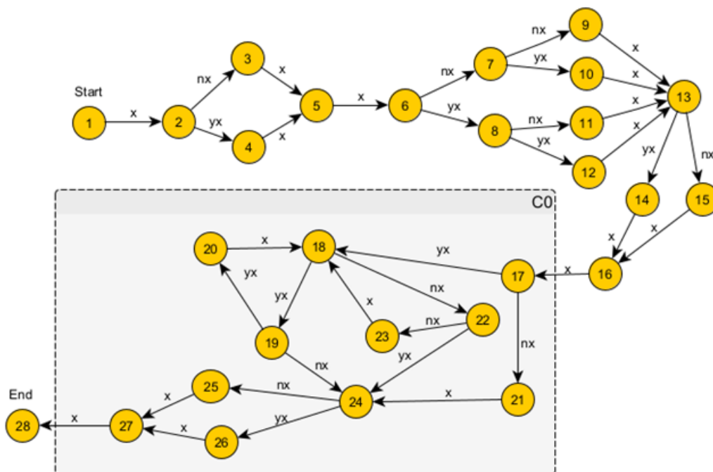
Рисунок 2 – Граф переходов состояний автоматной модели последовательного приложения L_{Seq} ; выделен участок C0, предназначенный для последующего клонирования при переходе к режиму SPMD (Single Program, Multiple Data)
