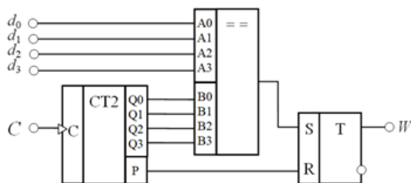
Рисунок 4 – Цифровой широтно-импульсный модулятор
