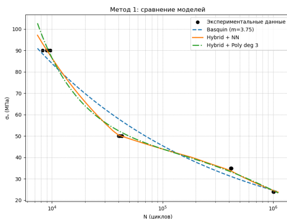
Рисунок 3 – Сравнение чистой S-N зависимости Баскина и гибридных моделей (NN и полиномиальной степени 3)
