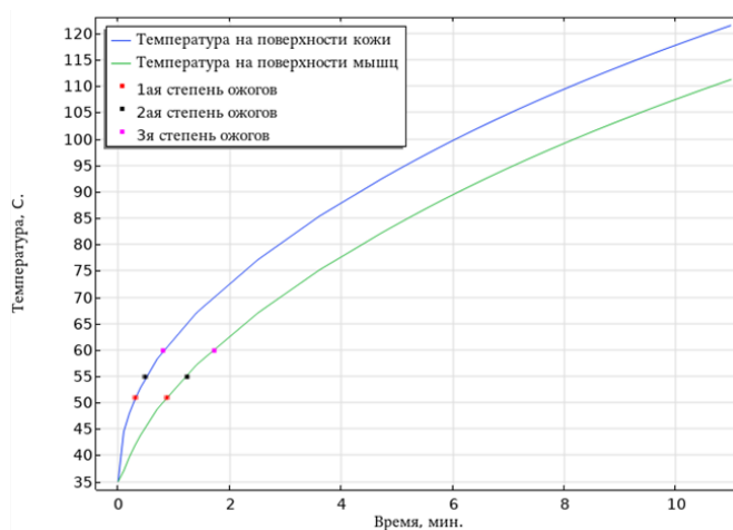
Рисунок 10 – Температура поверхности кожи и мышечной ткани от времени при нагреве от керамики
