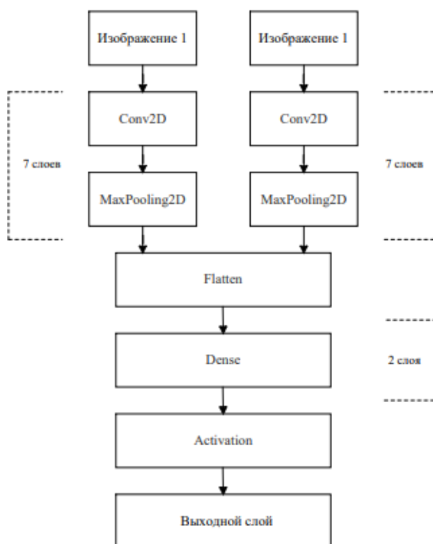
Рисунок 1 – Модель разработанной нейронной сети
