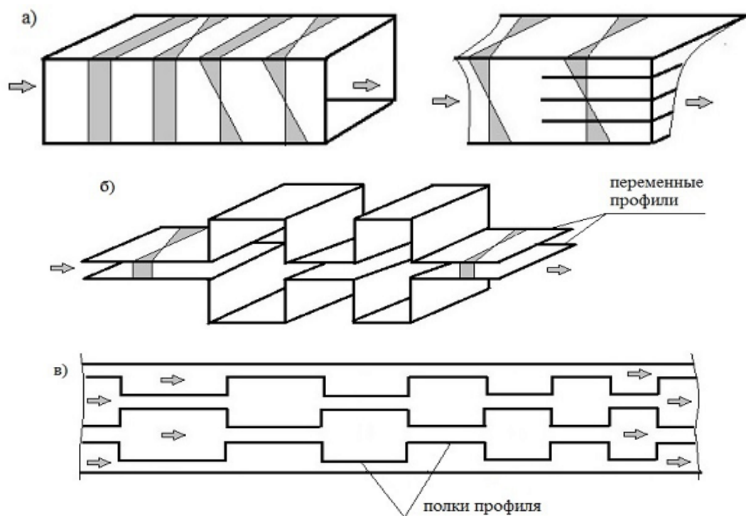
Рисунок 1 – Выполнение щелевого глушителя в магистральном воздуховоде: а – разделение воздуховода на щелевые каналы; б) компоновка щелевых расширительных камер; в) формирование различающихся щелевых каналов
