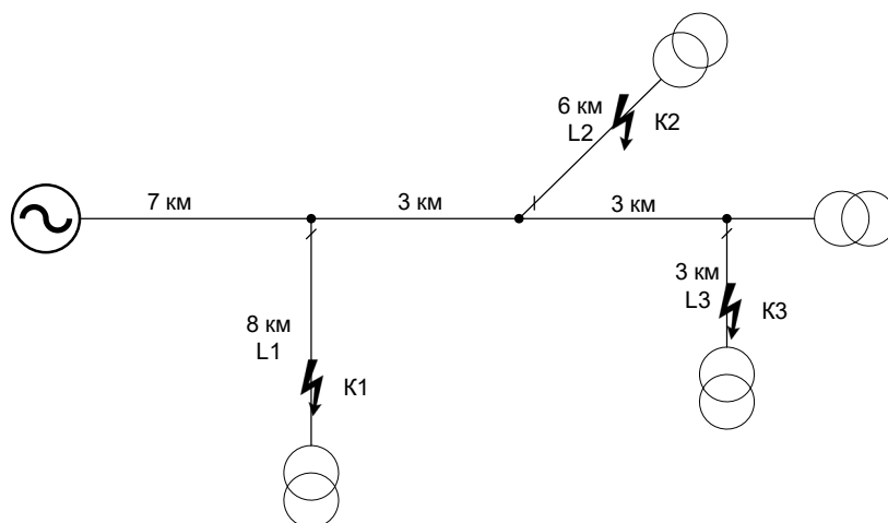
Рисунок 6 – Разветвленная распределительная электрическая сеть
