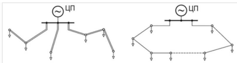
Рисунок 2 – Радиально-магистральная и замкнутая кольцевая конфигурация сети
