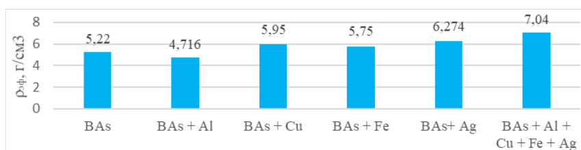
Рисунок 2 – Параметры плотности исследуемых композитных материалов
