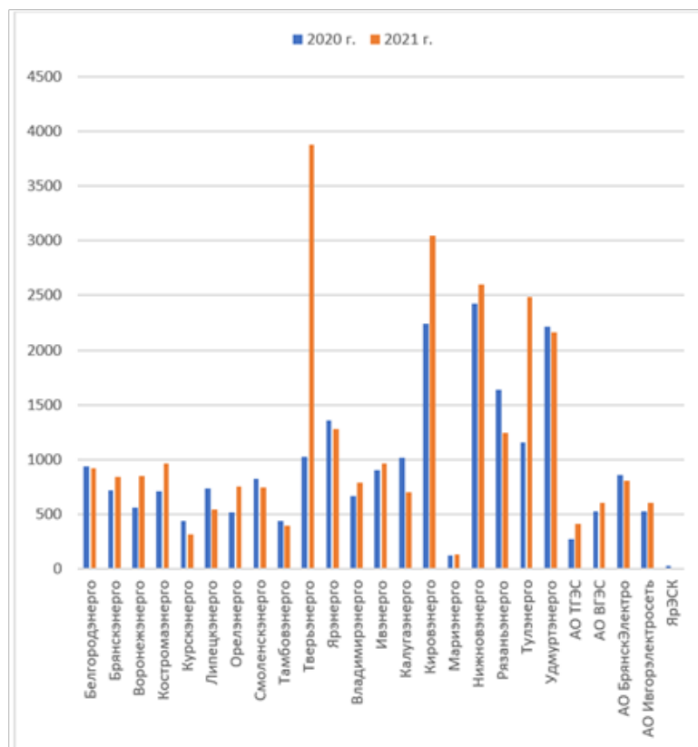
Рисунок 4 – Число аварийных отключений ВЛ 6-10 кВ ПАО «Россети»
