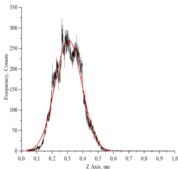
Рисунок 6 – Гистограмма распределения пор в матрице неорганического вяжущего, модифицированного 0,15 масс. % УНС
