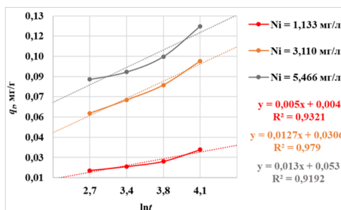
Рисунок 6 – Кинетические кривые в координатах уравнения Еловича
