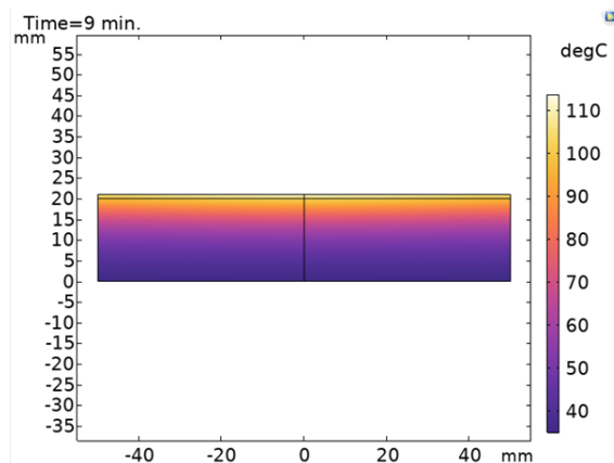
Рисунок 7 – Распределение температуры живой ткани в момент времени 9 минут (керамика)
