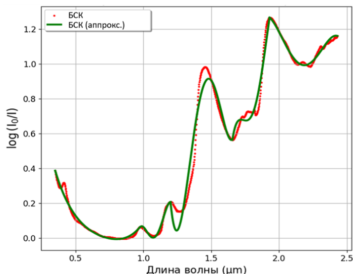
Рисунок 3 – Спектр поглощения для кожи белого кролика и его аппроксимация
