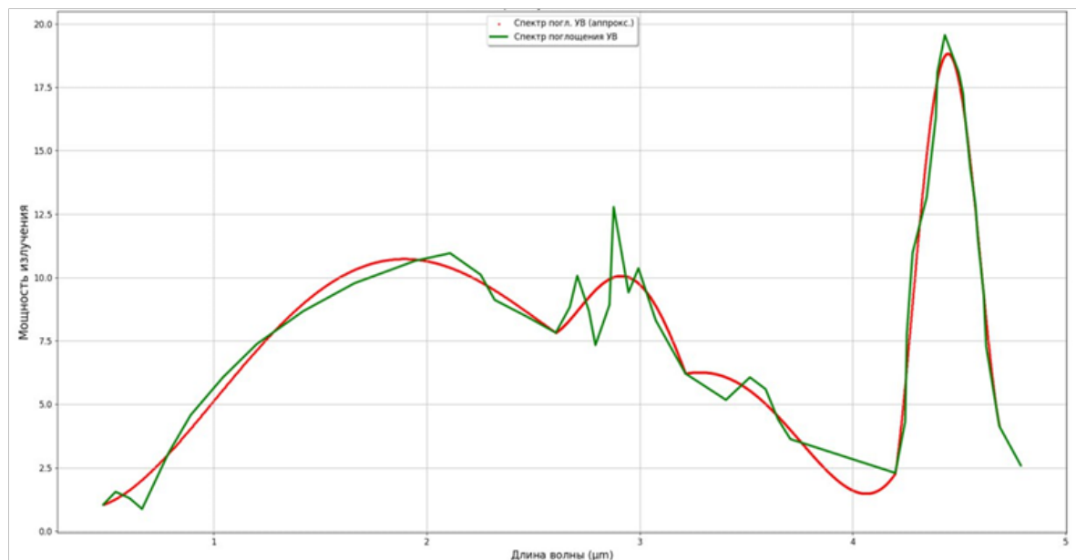
Рисунок 5 – Спектр излучения пламени углеводов
