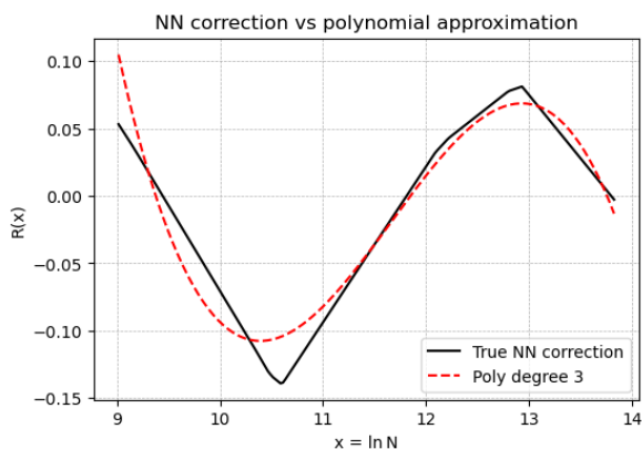
Рисунок 2 – Сравнение корректирующего слагаемого R(\ln N) и его полиномиальной аппроксимации
