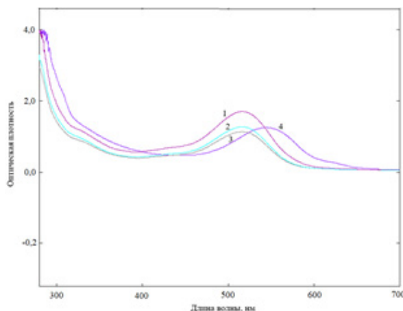
Рисунок 2 – УФ-спектры антоциановых экстрактов в зависимости от типа экстрагента и температуры экстрагирования (водой при 60 (1), 100 (2) и 25°C (3), 95% этиловым спиртом при 25°C (4))
