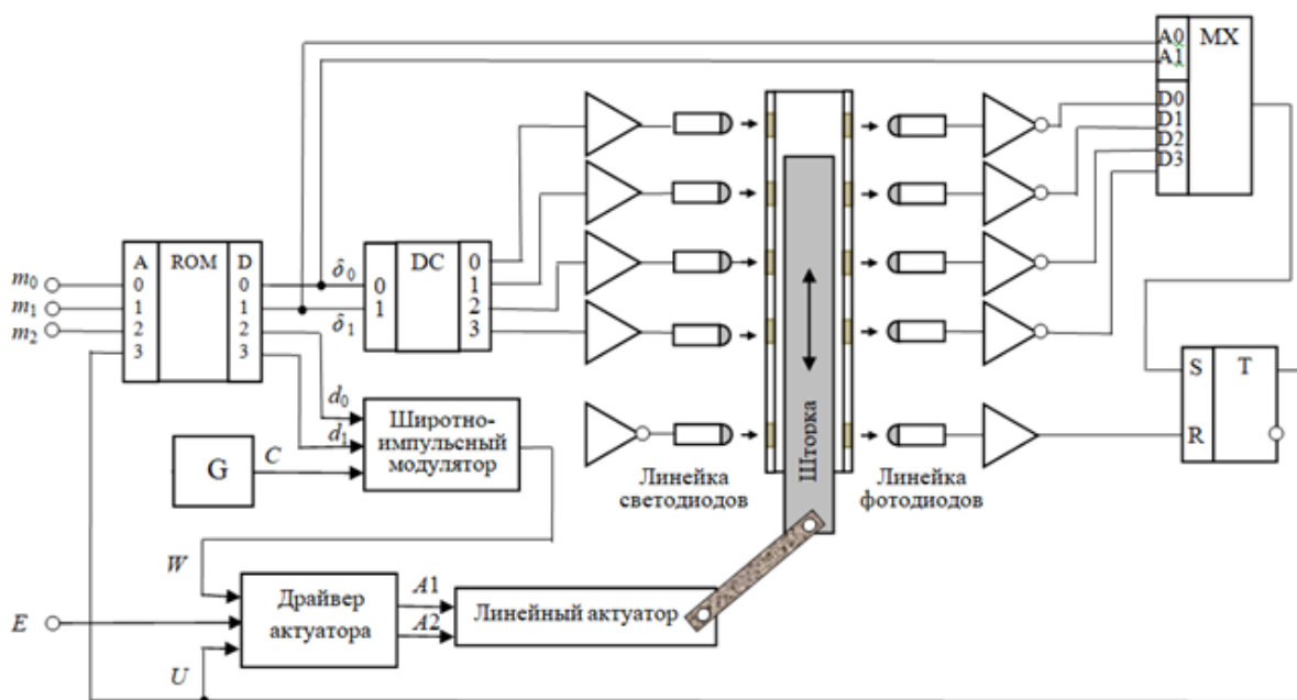
Рисунок 3 – Схема управления линейным актуатором
