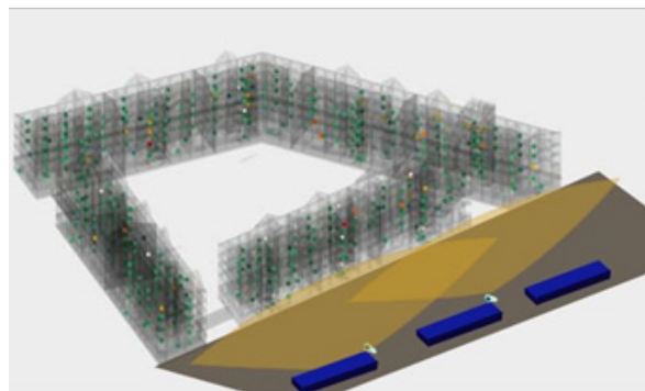
Рисунок 4 – Схема размещения смарт-видеокамер на участке строительной площадки ЖК «Пулковский дом»
