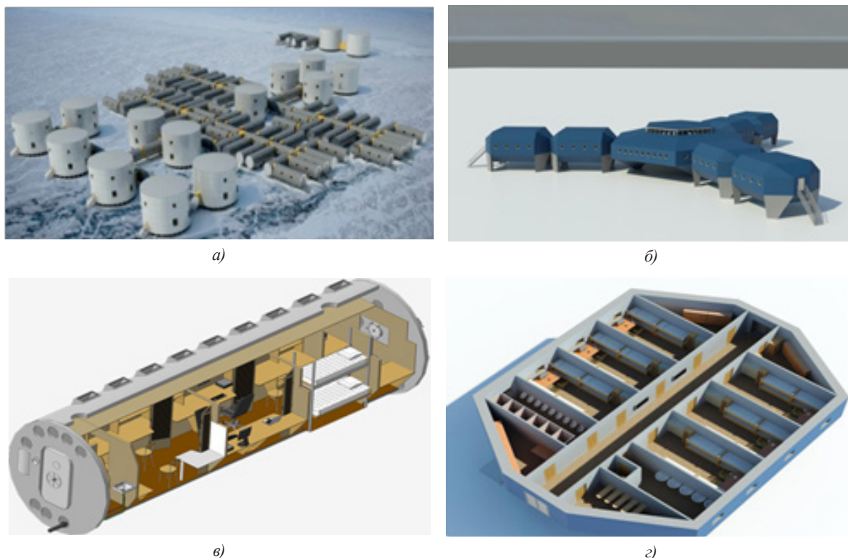
Рисунок 1 – Модульные объекты в АЗ (а, б) и виды модулей – ЦУБ (в) и октагонный (з) [14]
