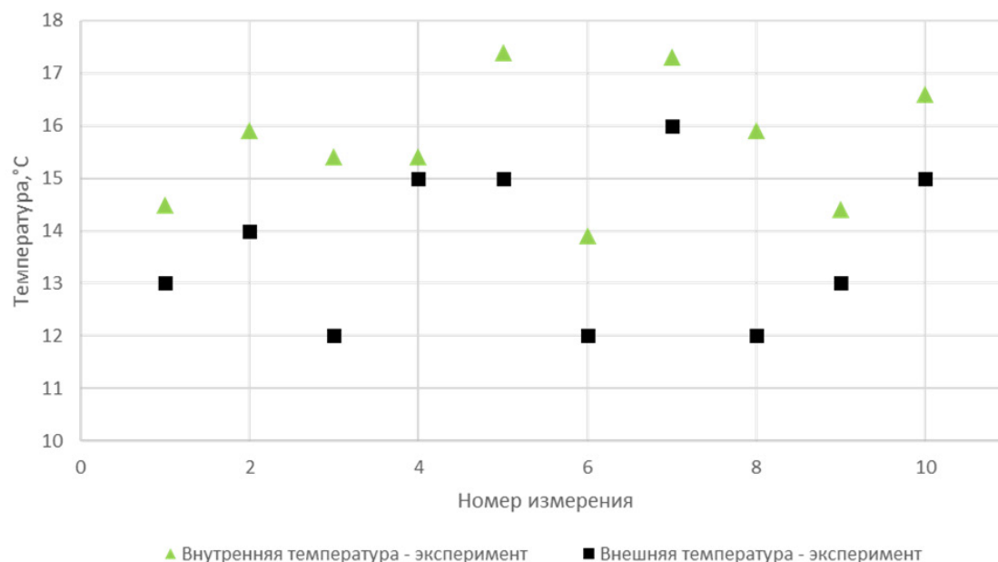
Рисунок 9 – Сравнение внешней и внутренней температуры по результатам экспериментальных исследований для холодного периода года
