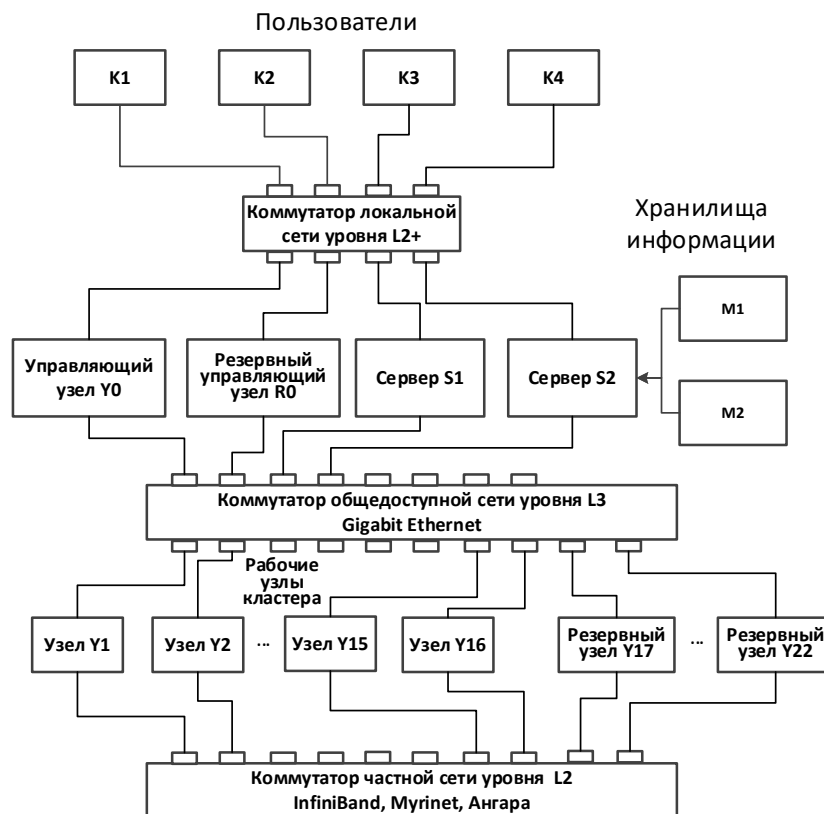
Рисунок 1 – Типовая архитектура вычислительного кластера, встроенного в инфраструктуру локальной вычислительной сети
