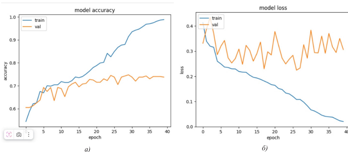
Рисунок 4 – График сходимости нейронной сети на спектральных представлениях
