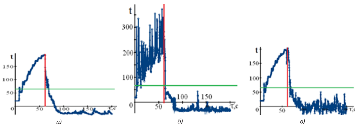
Рисунок 5 – Динамика температуры в модуле (рис. 1в) при продувке наружным воздухом с температурой минус 400С и скоростью V_B=10 м/с [34]: а – левая часть модуля, б – средняя часть, в – правая часть (здесь: t – температура у потолка, 0С; \tau – время, отсчитываемое от начала пожара, с; зелёная линия – болевой порог) [14]
