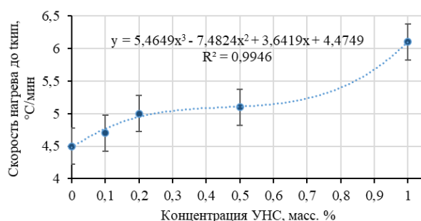
Рисунок 5 – Зависимость скорости нагрева до температуры кипения от концентрации УНС
