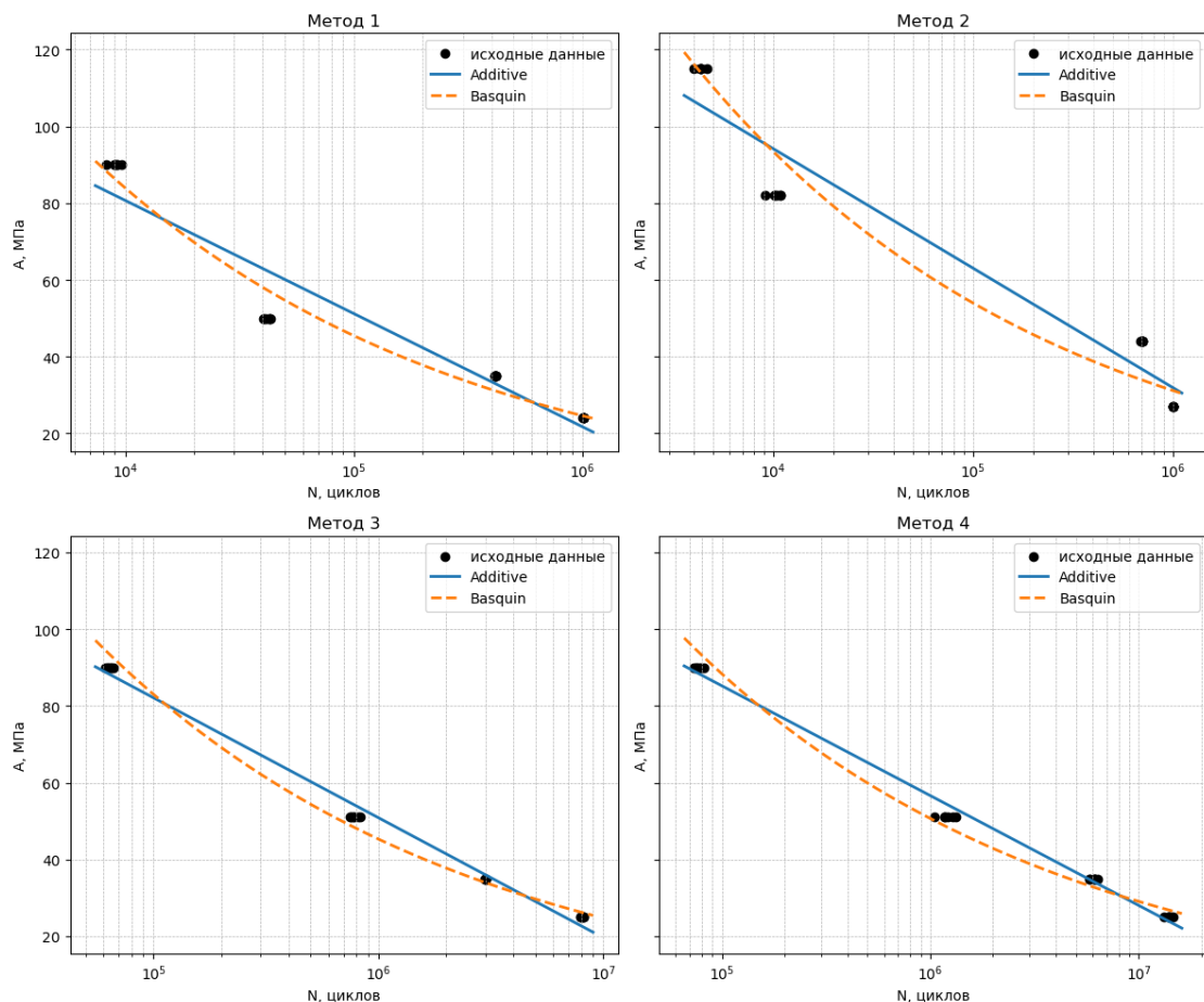
Рисунок 1 – ( S - N )-кривые для ремонтных технологий 1–4: аддитивная регрессия и модель Баскина
