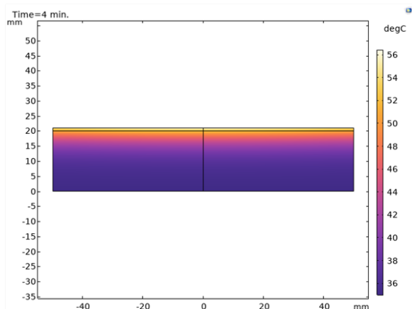
Рисунок 8 – Распределение температуры живой ткани в момент времени 4 минуты (УВ)
