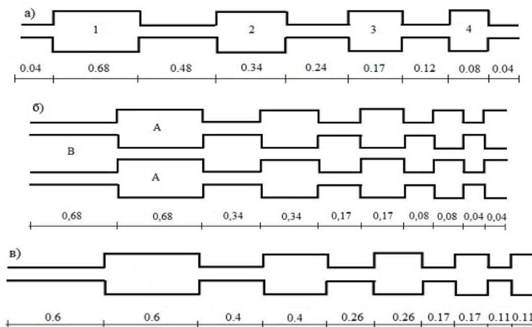
Рисунок 2 – Варианты щелевых устройств:
