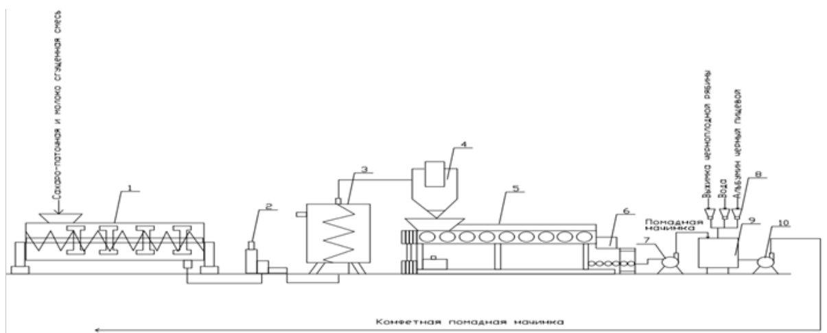
Рисунок 1 – Машинно-аппаратная схема получения помадной начинки с добавлением выжимок черноплодной рябины:
