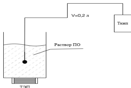
Рисунок 4 – Принципиальная схема процесса нагрева до температуры кипения
