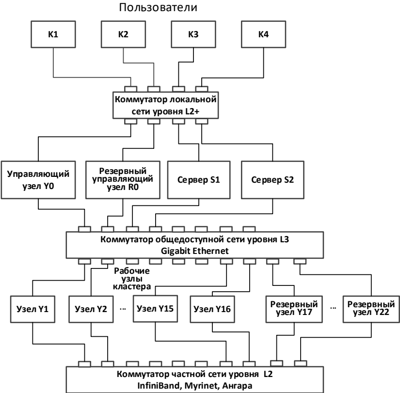
Рисунок 1 – Архитектура вычислительного кластера, встроенного в инфраструктуру локальной вычислительной сети
