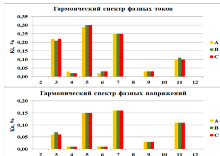
Рисунок 4 – Изменения коэффициентов гармонических искажений фазных токов и напряжений при износе подщипника синхронной электрической машины СД-13-34-8 на 10%
