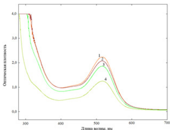
Рисунок 4 – УФ-спектры антоциановых экстрактов, выделенных 4% раствором пектиназы в течение 60 (1), 120 (2), 180) мин (3) и водным раствором без фермента (4)
