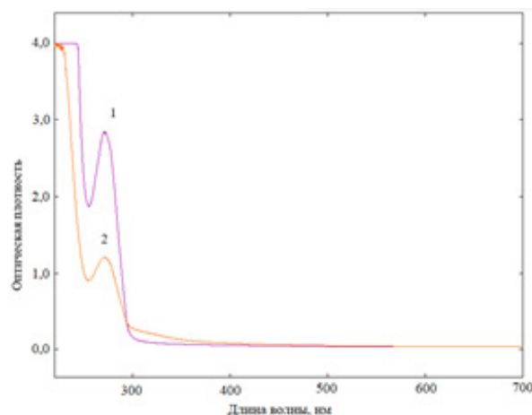
Рисунок 1 – УФ-спектры пектиновых растворов до (1) и после ферментативного гидролиза пектиназой (2)
