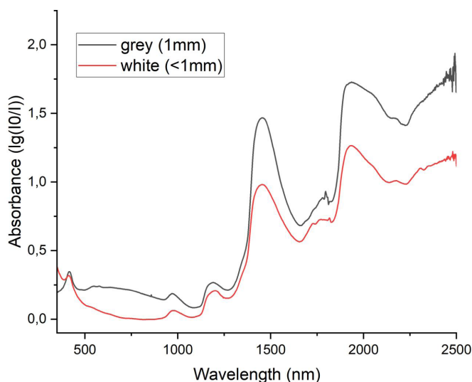
Рисунок 1 – Спектр поглощения для кожи белого и серого кролика
