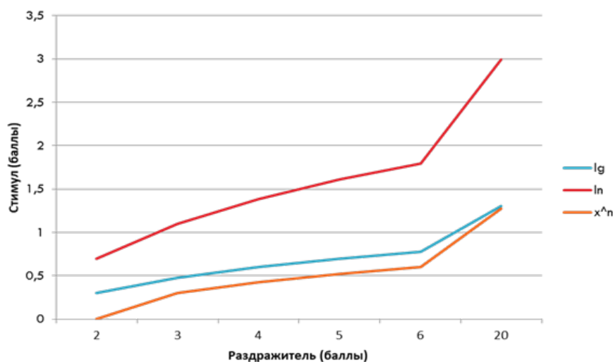
Рисунок 1 – Вид графиков изменения стимула от изменения интенсивности раздражителя при использовании функций \lg , \ln , x^n
