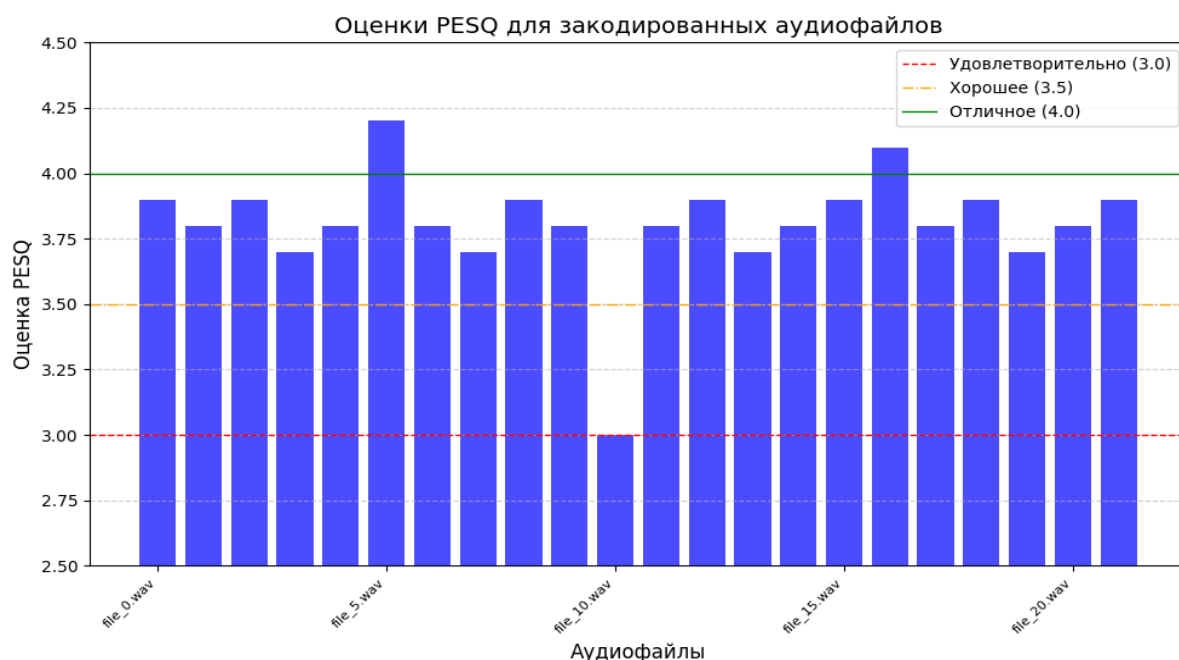
Рисунок 3 – Оценки PESQ
