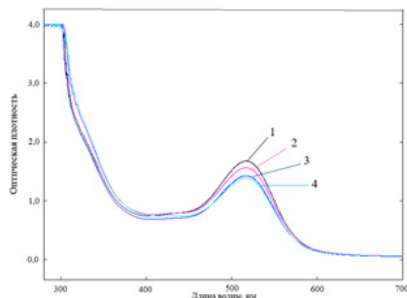
Рисунок 3 – УФ-спектры антоциановых экстрактов в зависимости от концентрации пектиназы (4% (1), 3% (2), 2% (3), 1% (4)) в условия экстракции 60 мин при температуре 50°C, pH среды 4,01
