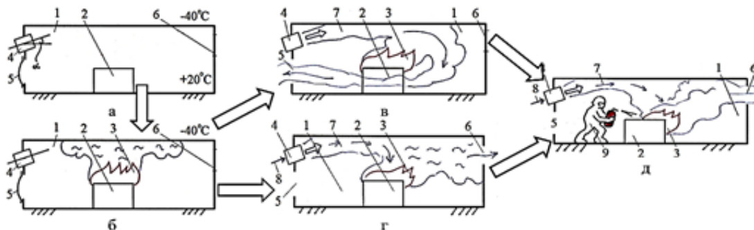
Рисунок 3 – Этапы тушения пожара в арктическом модуле посредством продувки наружным низкотемпературным воздухом с дозированной подачи снега/воды:
