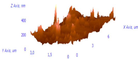
Рисунок 2 – Структура защитного материала 2-D а) без УНС б) с УНС
