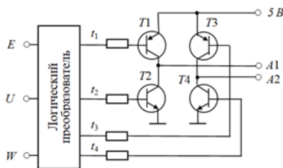
Рисунок 5 – Драйвер актуатора
